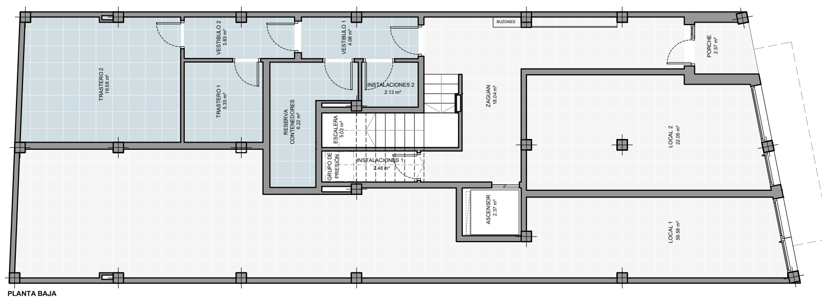
PLANTA BAJA
